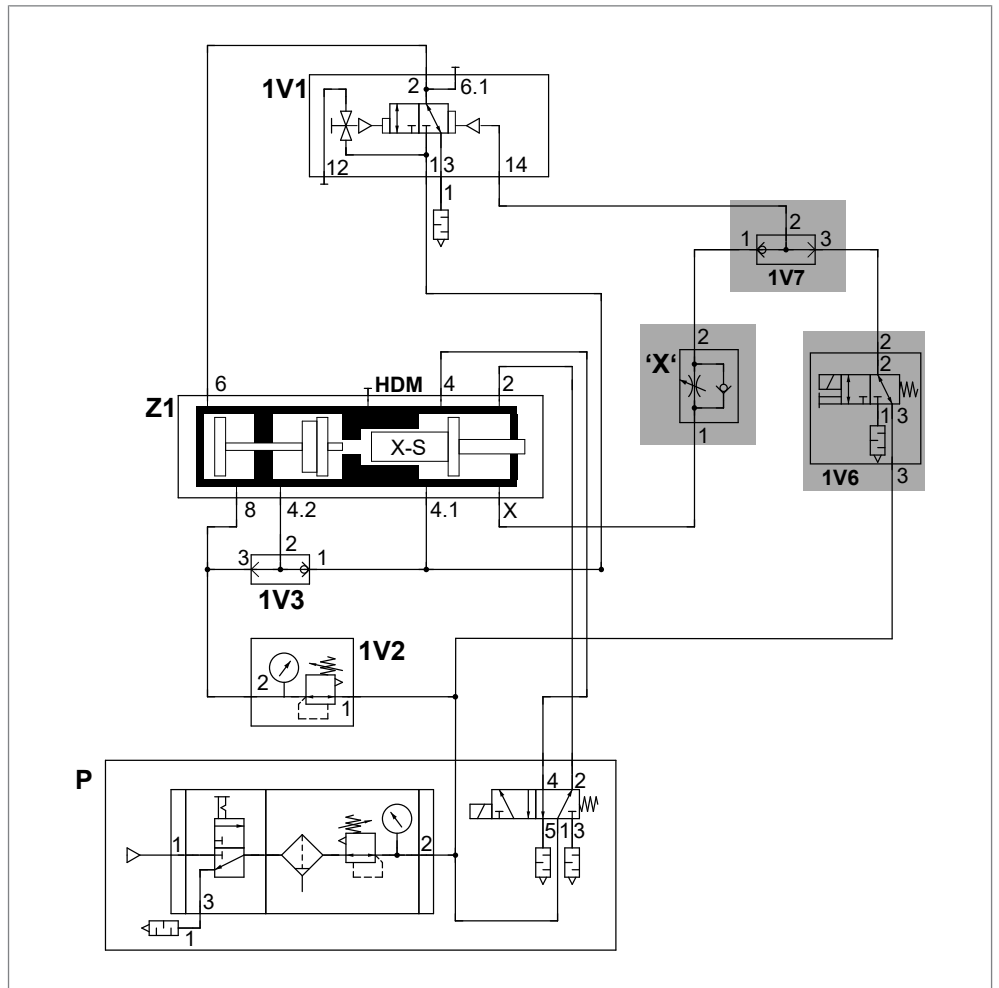
Fig. 8 Liberación de la carrera de trabajo externa (grupo constructivo ZKHF)
