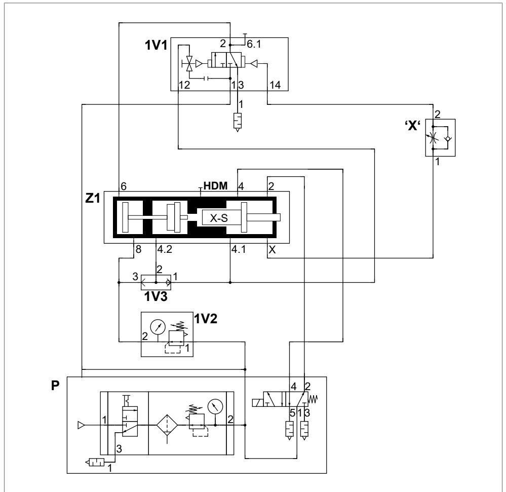
Fig. 9 Alimentación externa de la carrera de potencia (opcional)
