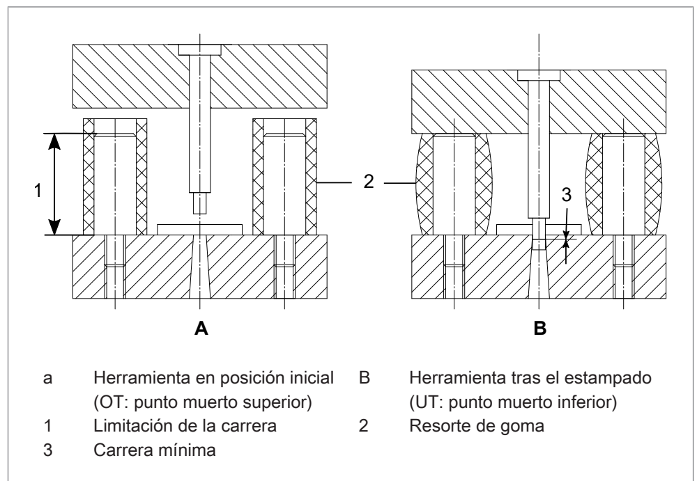
Fig. 2 Limitación de la carrera en la herramienta
