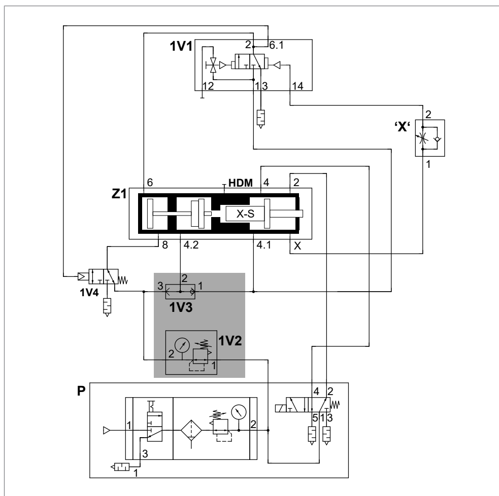
Fig. 3 Accionamiento del proceso de presión dinámica con resorte neumático y soporte de carrera rápida y desconexión del soporte neumático en la línea de la carrera de potencia (line-X, X-75 y X-100)
